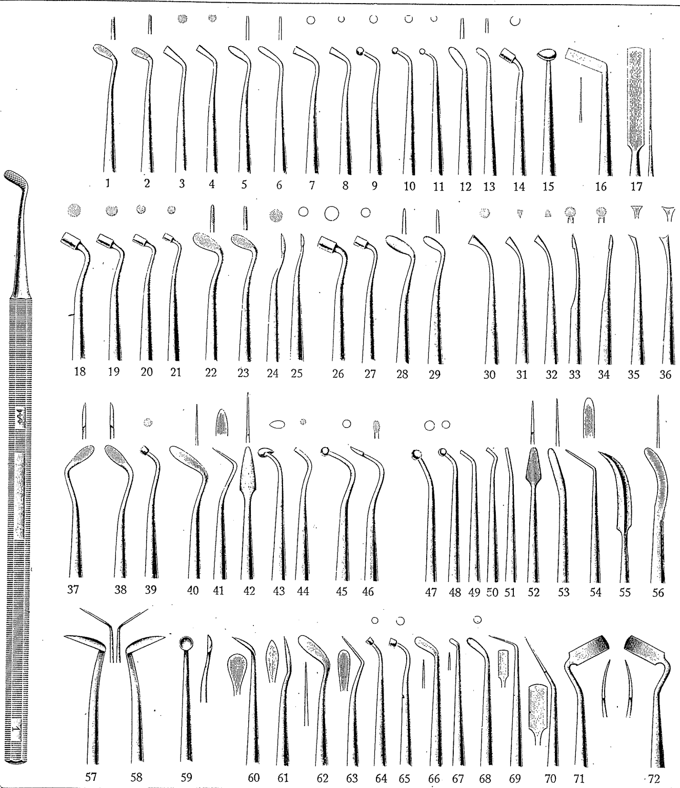
D/.. 3362 Instrumente für Amalgam, Zement und Guttapercha, Fig. 1—72
